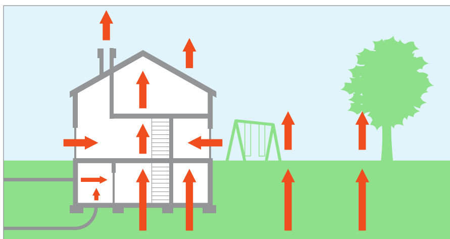
L'aria del suolo contenente radon penetra all'interno dell'edificio o nell'aria.
